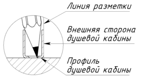
Вид А М(2:1.5) Повернуто
